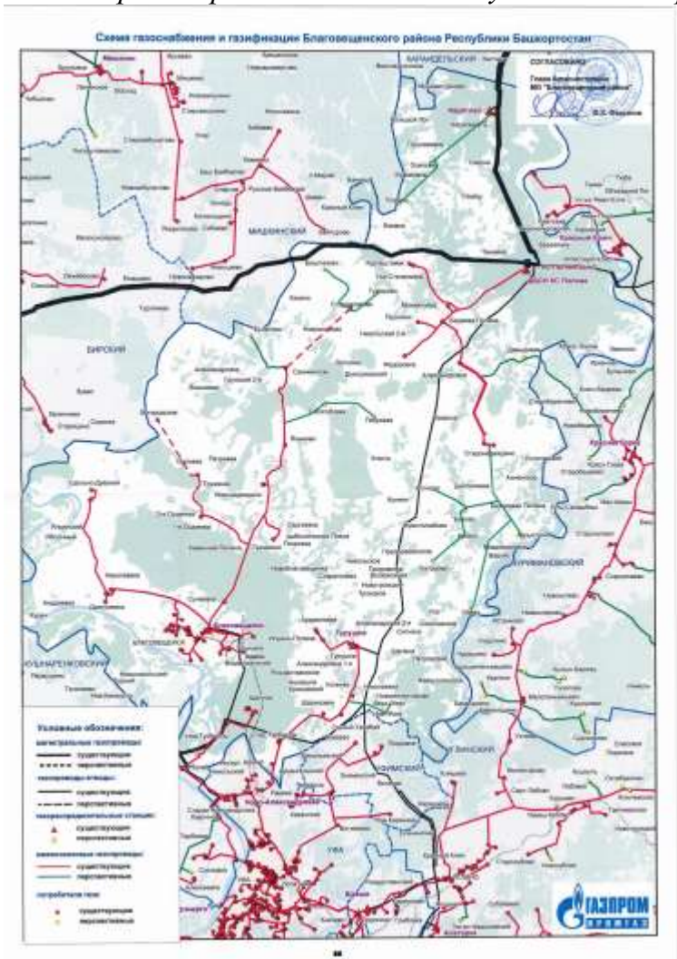
Рис.: Газотранспортная система муниципального района Благовещенский район Республики Башкортостан.
